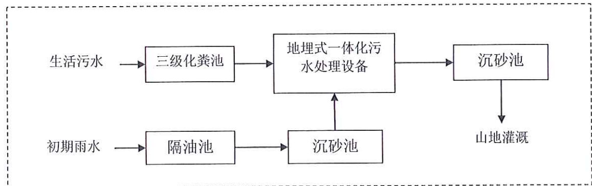
图 3-1 项目污水处理工艺流程
